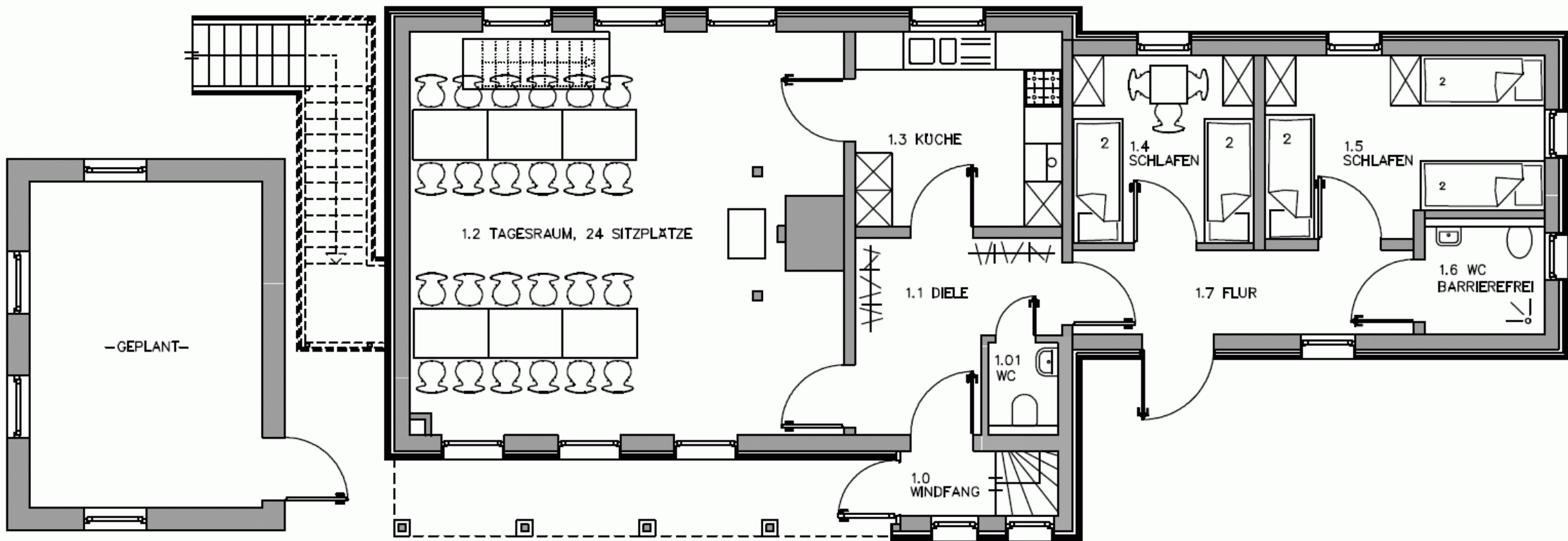
GRUNDRISS ERDGESCHOSS
